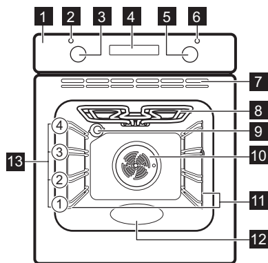
1 Kontrollpanel
