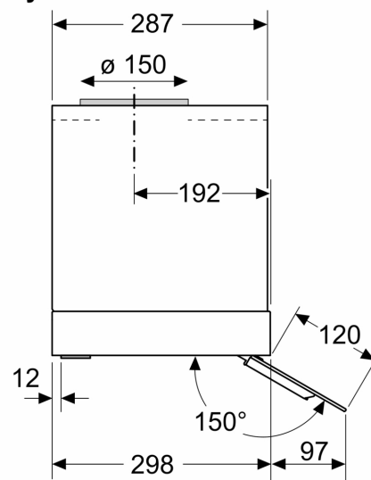
Mått i mm Sidovy
